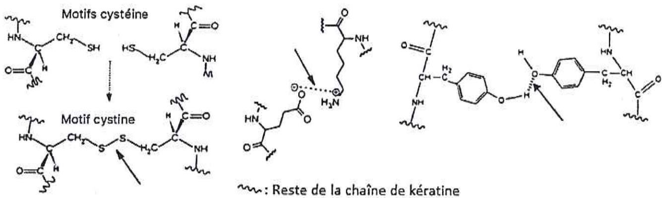
Figure 2 – Liaisons et interactions maintenant les différentes molécules de kératine entre elles
