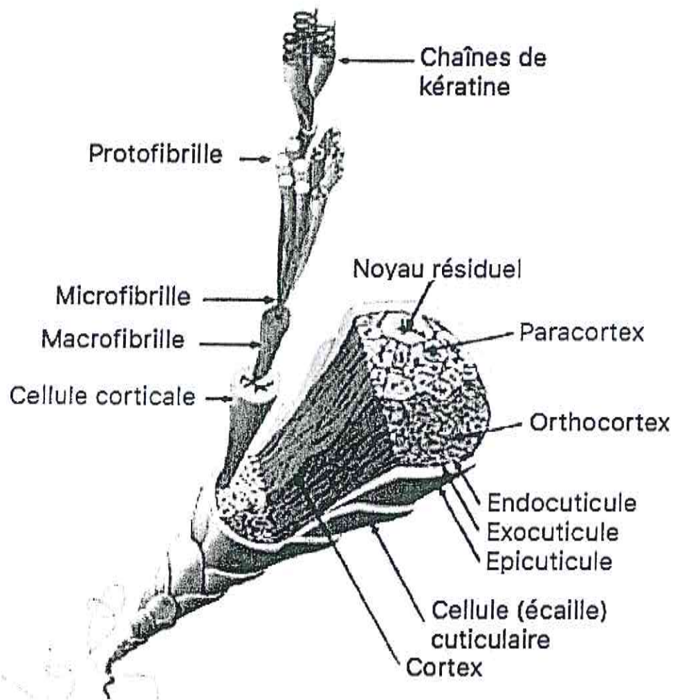
Figure 1 – Schéma de la fibre capillaire humaine.
